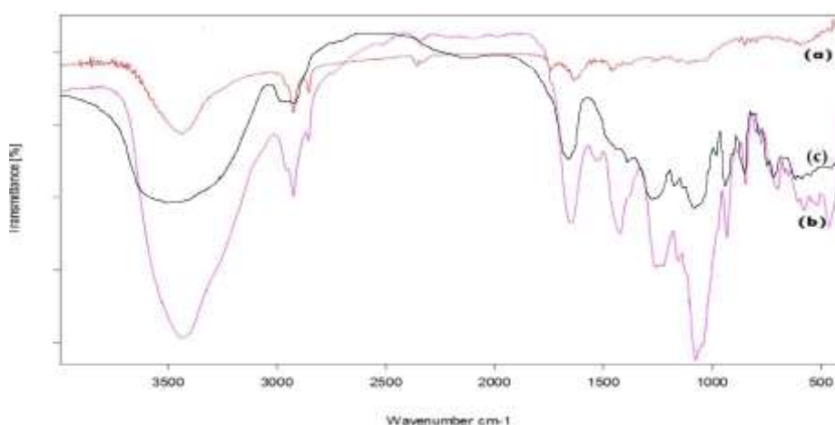
شکل ۱. طیف FTIR کاراژینان استخراج شده از ماکروجلبک H. flagelliformis تیمار آلكالی (a)، بدون تیمار (b) در مقایسه با کاراژینان تجاری (c).
